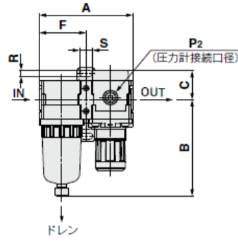
AC20B-D
