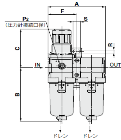
AC30D-D
