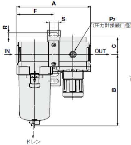
AC40B-D~AC60B-D
