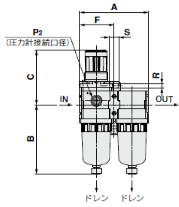
AC20D-D
