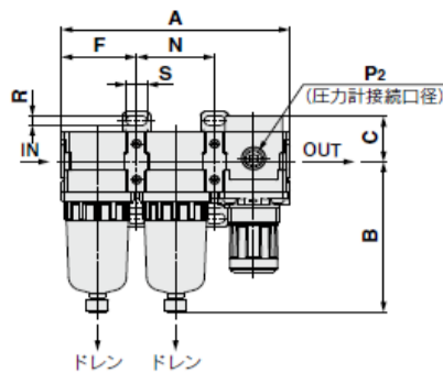
AC20C-D
