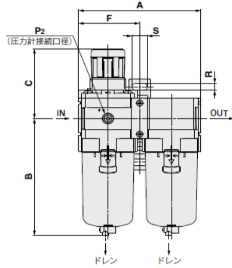
AC40D-D
