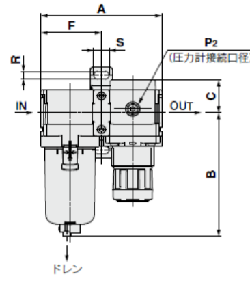
AC30B-D
