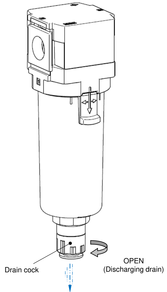
AFG30-D/ AFG40-D: Auto drain
